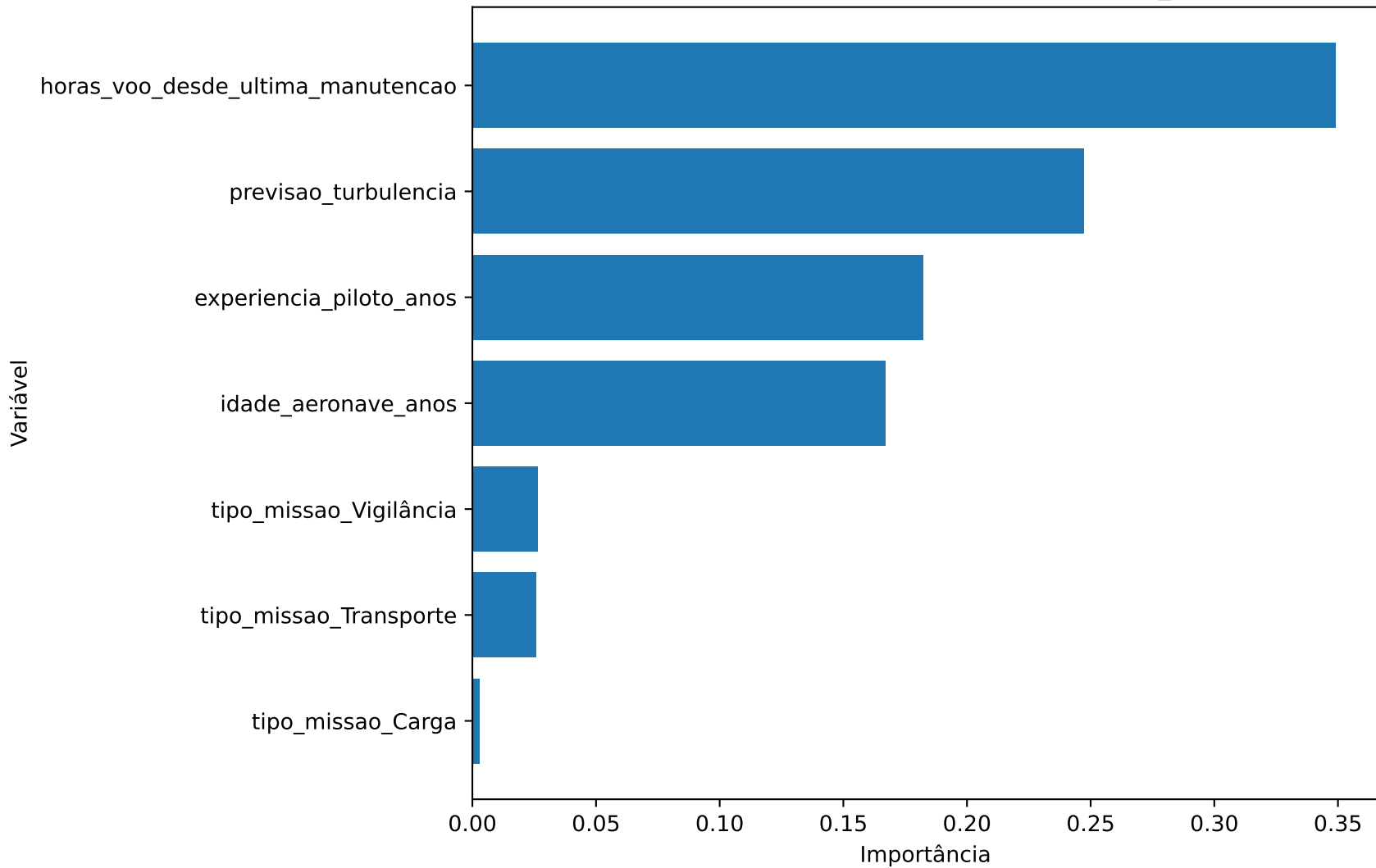
Top variáveis mais importantes — random_forest
